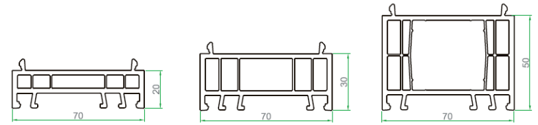
57054
